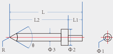
Diamond Stylus
