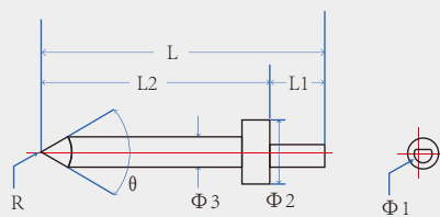
Tapered Stylus
